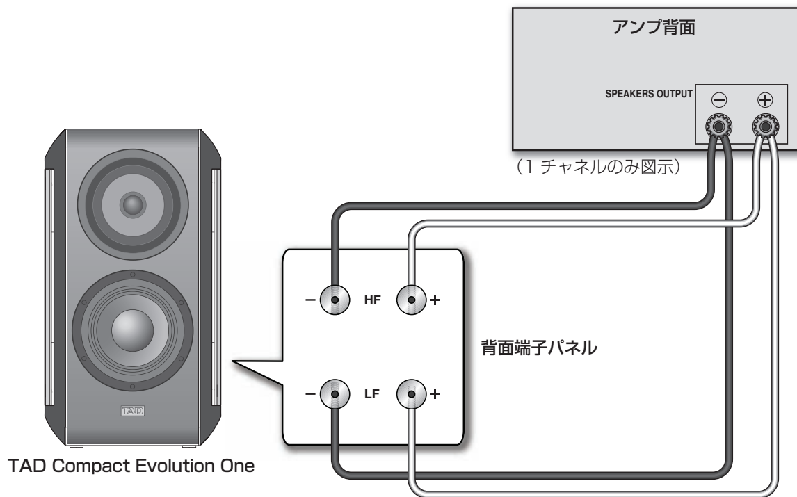
第 3 図 : TAD Compact Evolution One のバイワイヤリング接続
