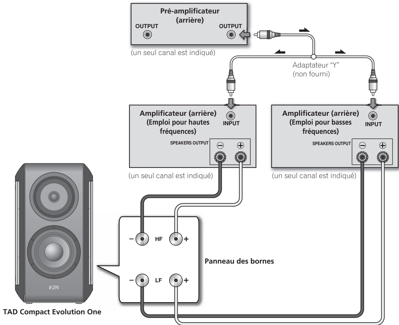
Figure 5. Connexion d'une enceinte TAD Compact Evolution One en un circuit à bi-amplification horizontale
