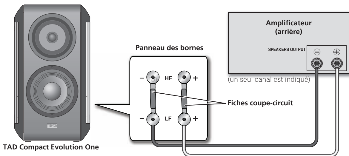
Figure 2. Connexion d'une enceinte TAD Compact Evolution One en un circuit unifilaire
