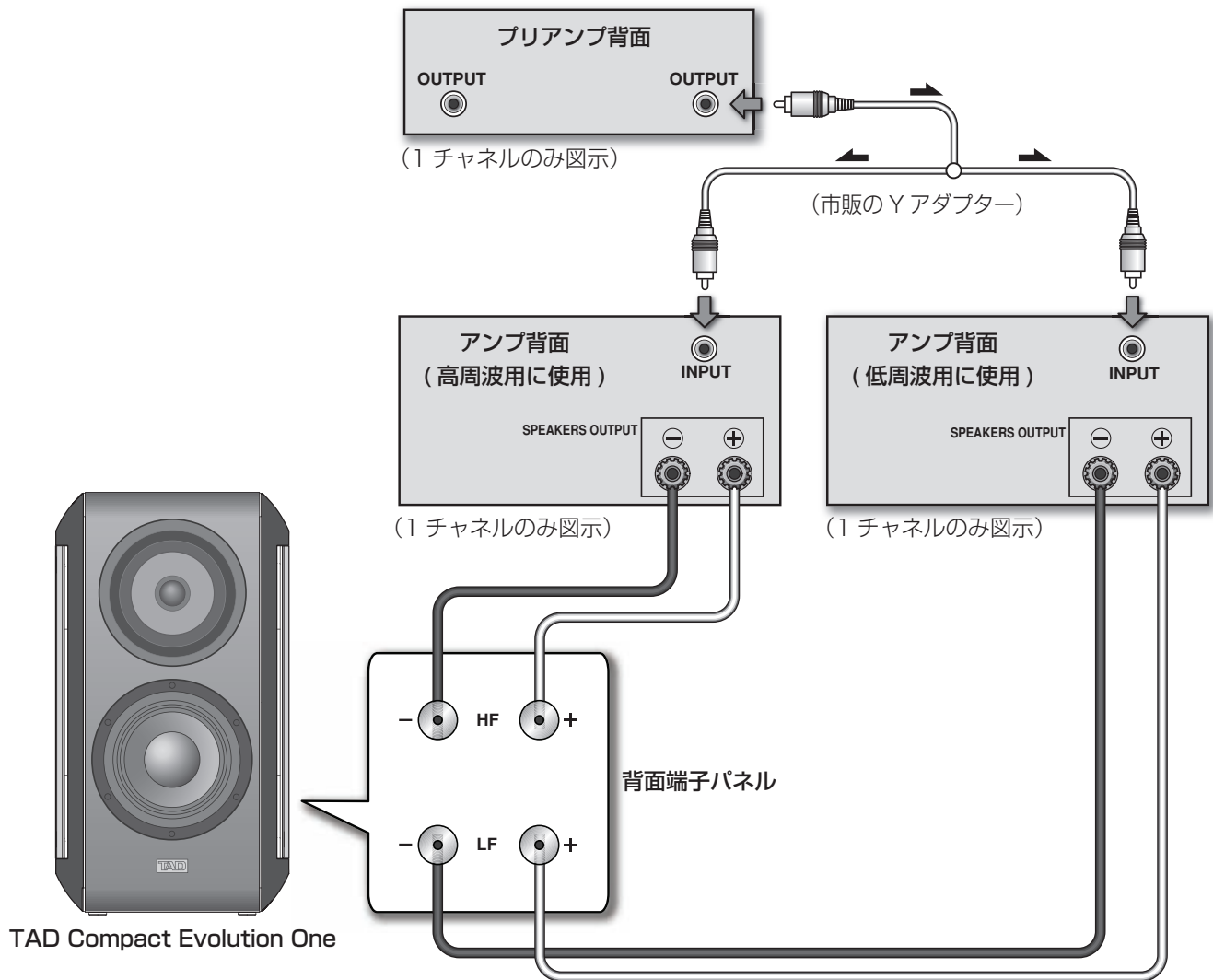
第 5 図 : TAD Compact Evolution One の 水平バイアンプシステム接続
