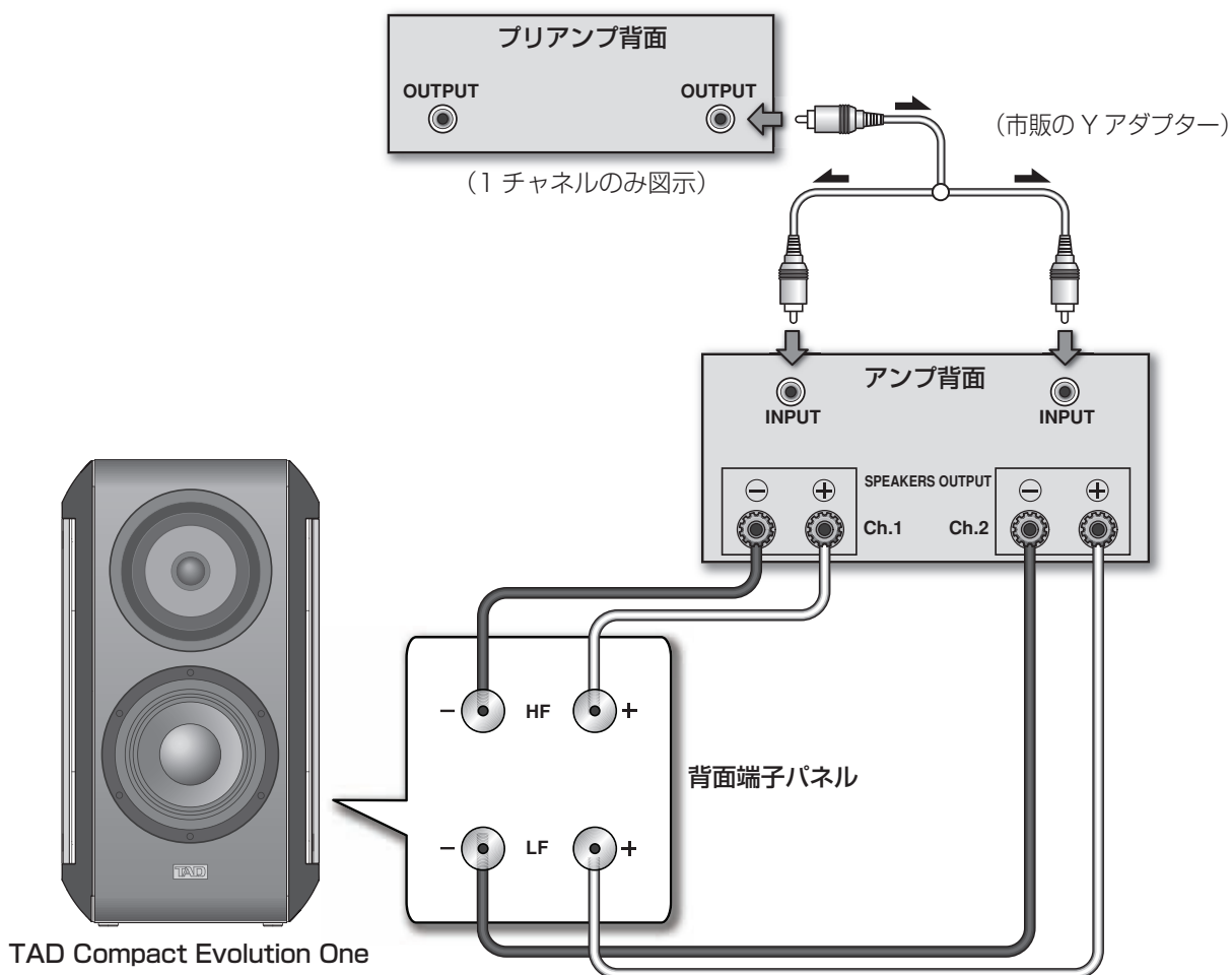
第4図：TAD Compact Evolution Oneのパーティカルバイアンプシステム接続
