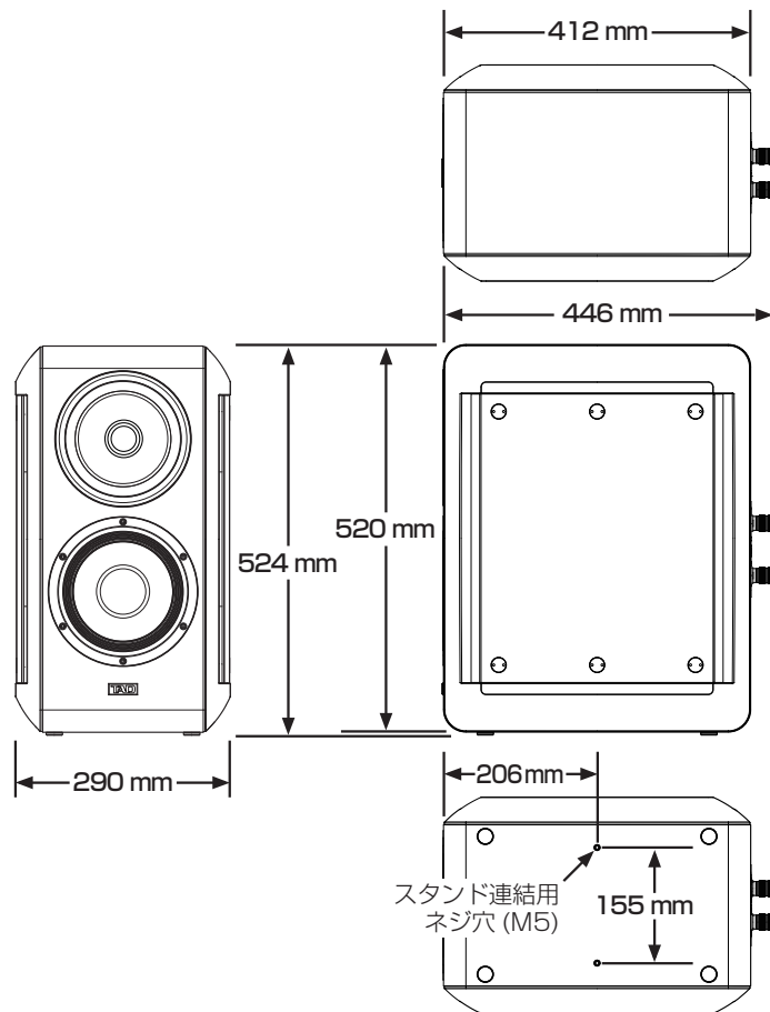
第 6 図：TAD Compact Evolution One スピーカーシステムの外形寸法
