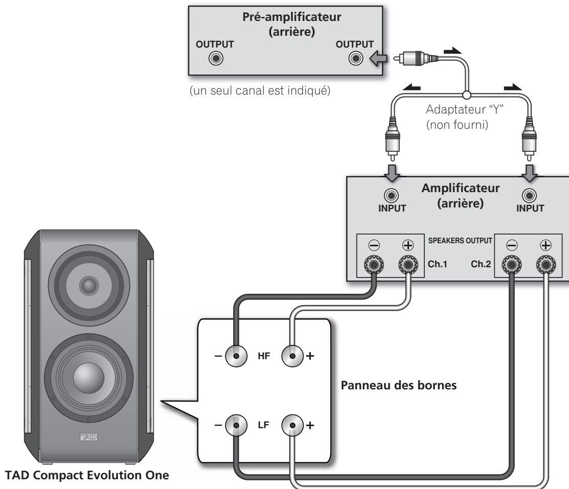
Figure 4. Connexion d'une enceinte TAD Compact Evolution One en un circuit bifilaire vertical
