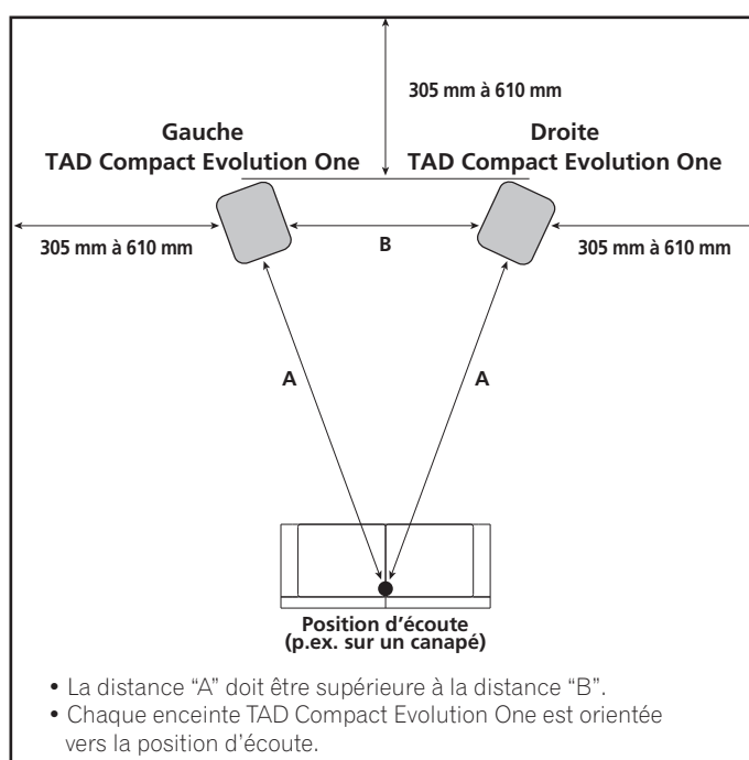
Figure 1. Emplacement d'une paire d'enceintes TAD Compact Evolution One pour une écoute en stéréo
