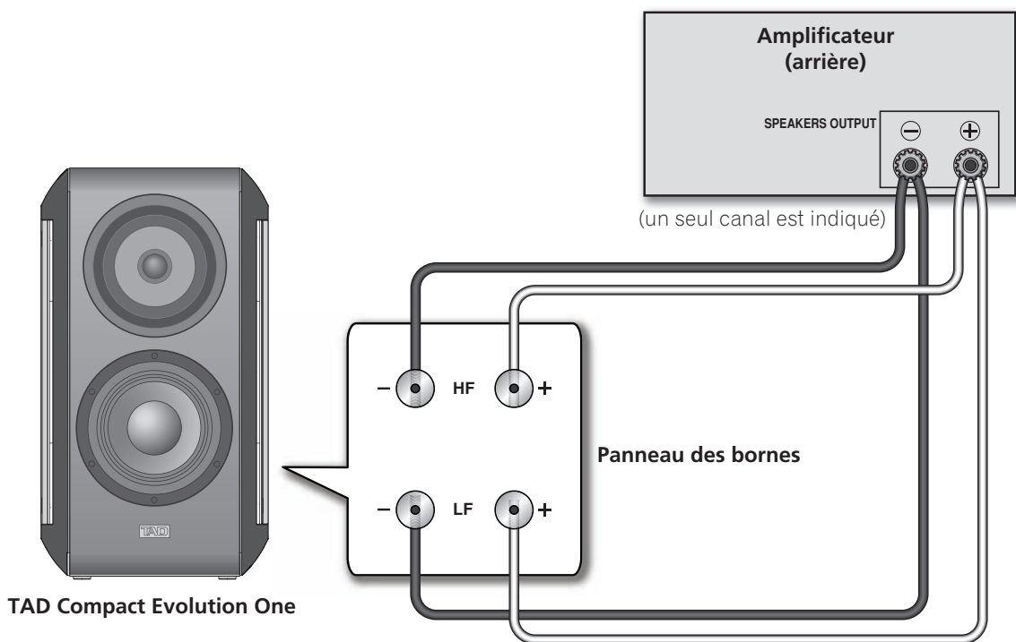
Figure 3. Connexion d'une enceinte TAD Compact Evolution One en un circuit bi-filaire
