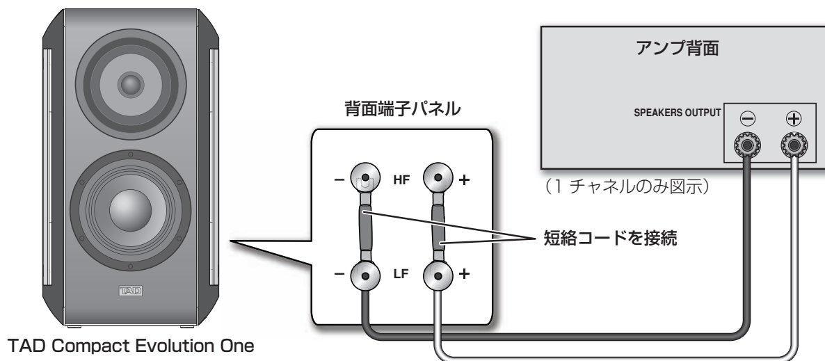
第 2 図 : TAD Compact Evolution One の シングルワイヤリング接続
