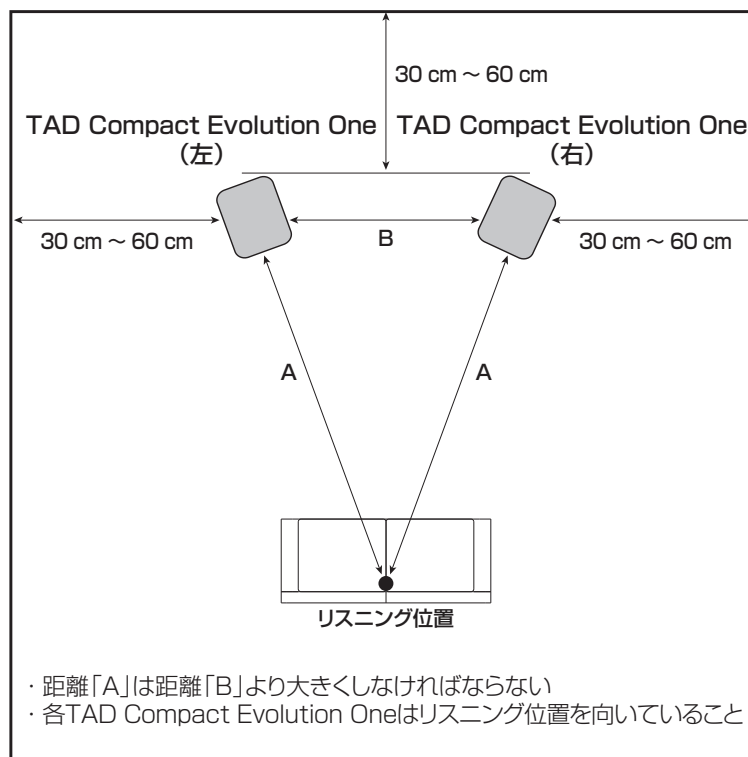
第1図：TAD Compact Evolution Oneの2チャンネルセッティング例
