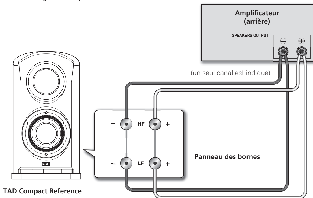
Figure 8. Connexion d'une enceinte TAD Compact Reference en un circuit bi-filaire
