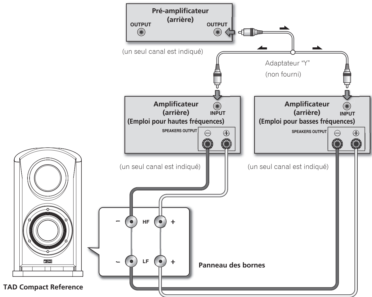
Figure 10. Connexion d'une enceinte TAD Compact Reference en un circuit bi-amplification vertical
