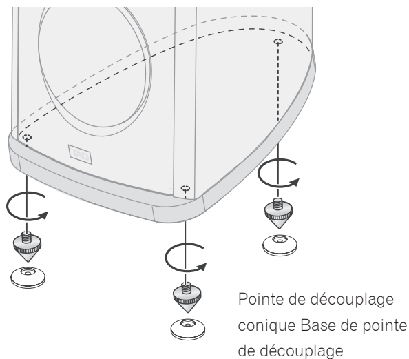
Figure 4 : Mise en place des pointes de découplage sur le fond de l'enceinte TAD Compact Reference
