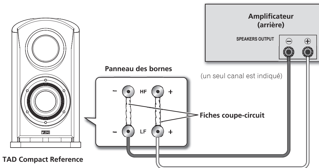
Figure 7. Connexion d'une enceinte TAD Compact Reference en un circuit unifilaire
