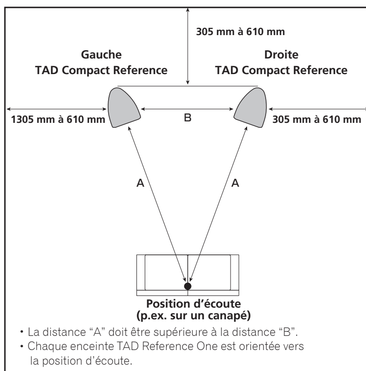
Figure 6. Emplacement d'une paire d'enceintes TAD Compact Reference pour une écoute en stéréo
