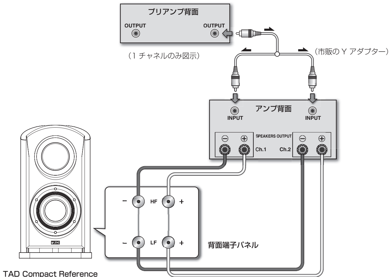
第 9 図 : TAD Compact Reference の バッチカルバイアンプシステム接続
