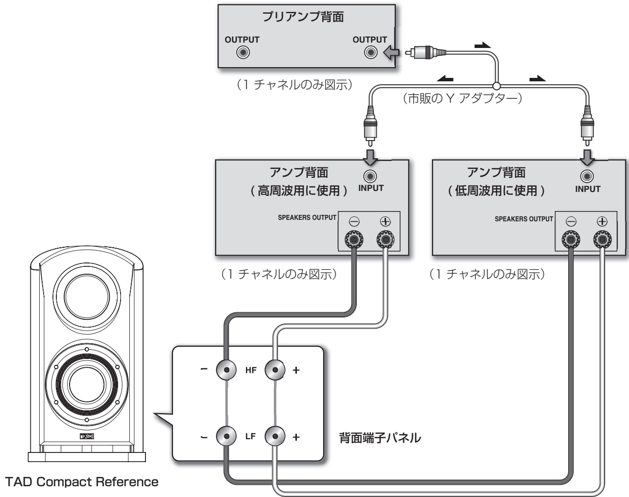
第 10 図：TAD Compact Reference の 水平バイアンプシステム接続
