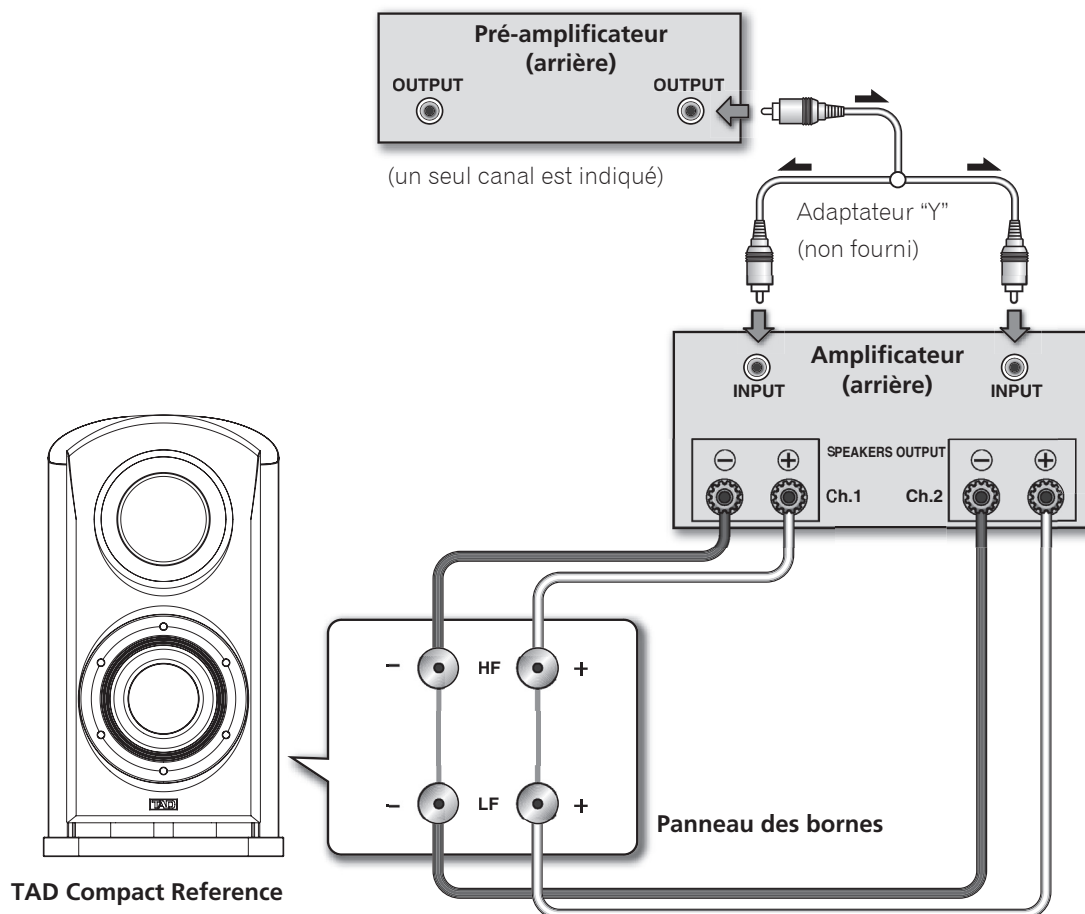
Figure 9. Connexion d'une enceinte TAD Compact Reference en un circuit bifilaire vertical
