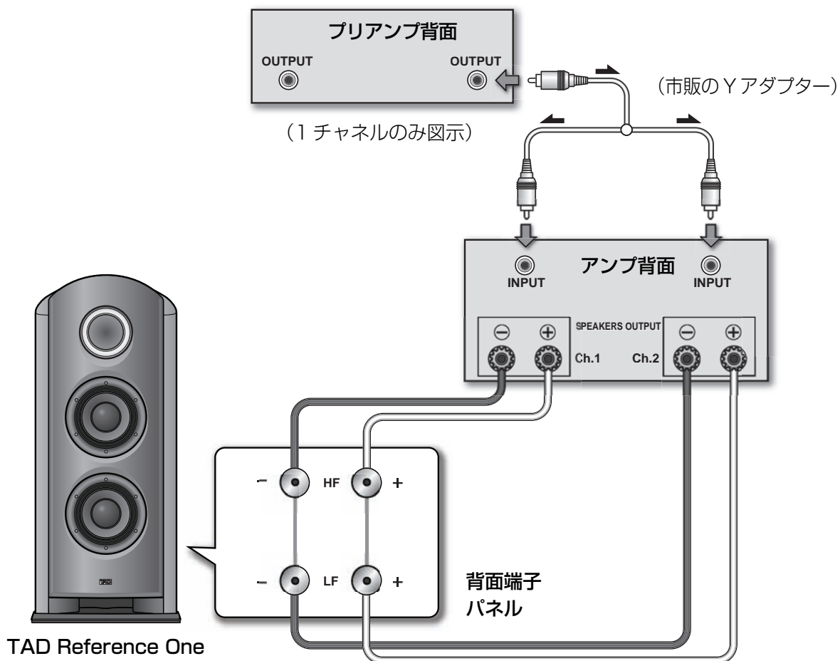
第10図：TAD Reference Oneの バーチカルバイアンプシステム接続
