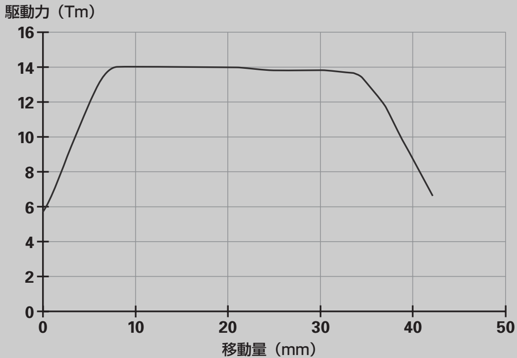
第4図：TAD Reference One ウーファーの変位（移動量）－駆動力特性
