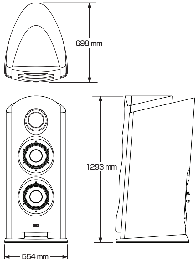
第 12 図 : TAD Reference One スピーカーシステムの外形寸法
