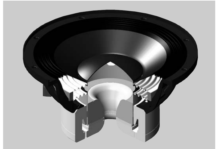
第3図：TAD Reference One のウーファー
