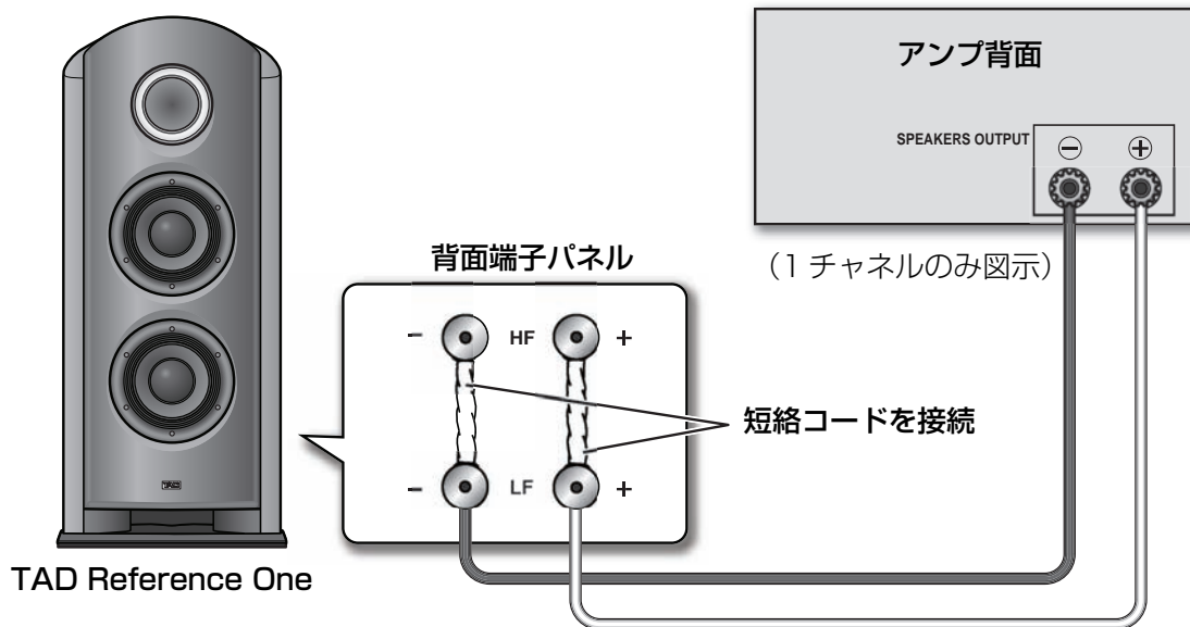
第8図：TAD Reference Oneの シングルワイヤリング接続
